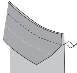
Piqûre I au point droit à la machine à coudre
