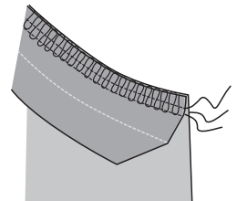
Piqûre I à la surjeteuse
